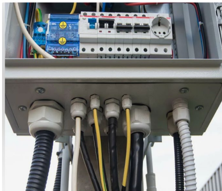
Герметизация кабеля СИП
