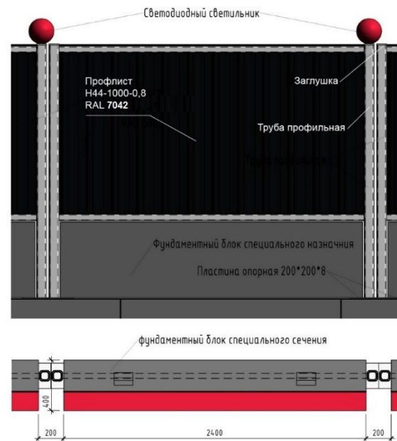
Ограждение с навесом тип 3 АН
